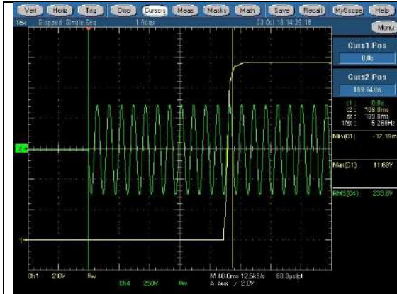
264V +12Vsb max CH1:+12Vsb, CH4:Vin
