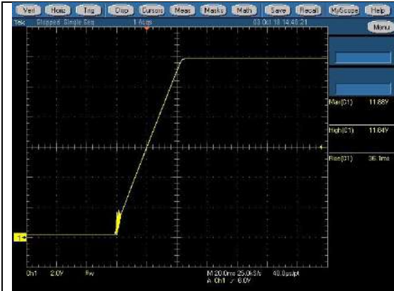
90V +12V max CH1:+12V
