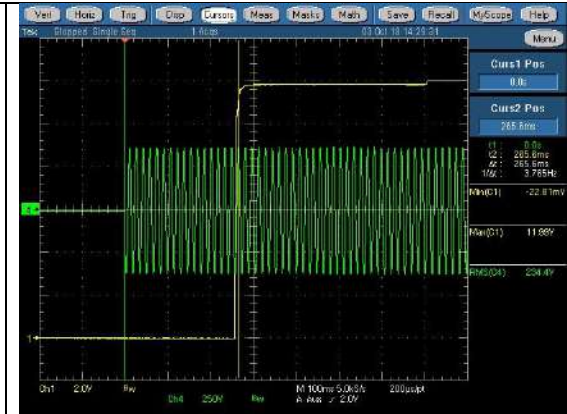
264V +12Vsb min CH1:+12Vsb, CH4:Vin
