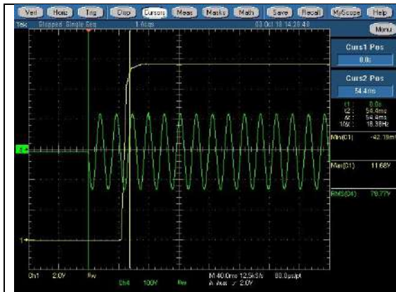
90V +12Vsb max CH1:+12Vsb, CH4:Vin
