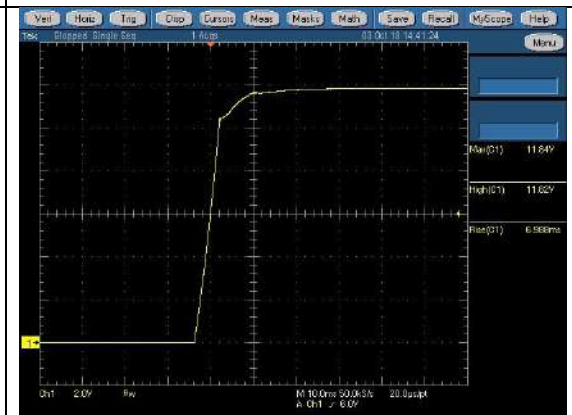
90V +12Vsb min CH1:+12Vsb
