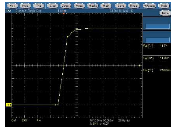
90V +12Vsb max CH1:+12Vsb
