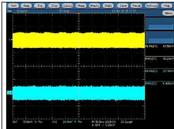
90Vac/47Hz Max Load CH1: +12V, CH2: +12Vsb
