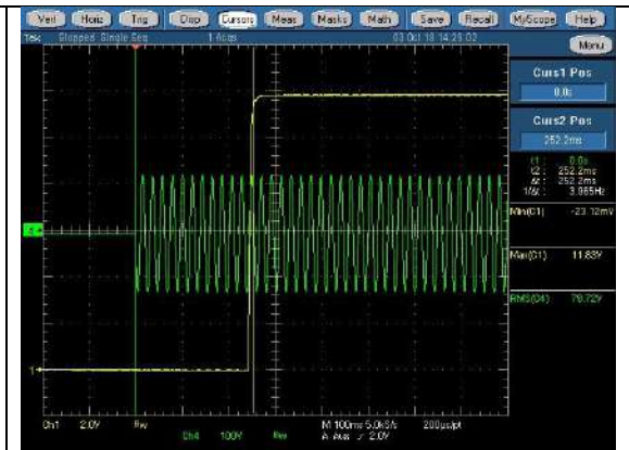
90V +12Vsb min CH1:+12Vsb, CH4:Vin
