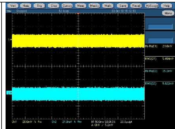
90Vac/47Hz Min Load CH1: +12V, CH2: +12Vsb
