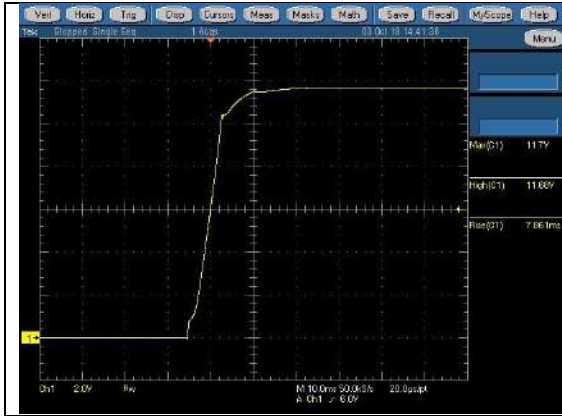
264V +12Vsb max CH1:+12Vsb
